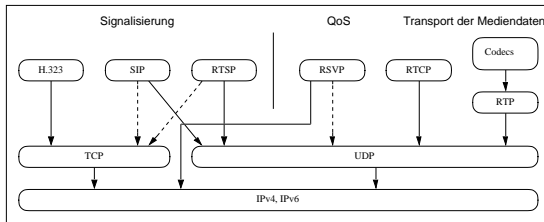
Abbildung 1: Zusammenwirken der Protokolle
