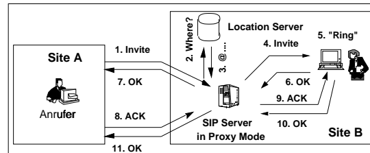
Abbildung 3: SIP-Gesprächsaufbau
