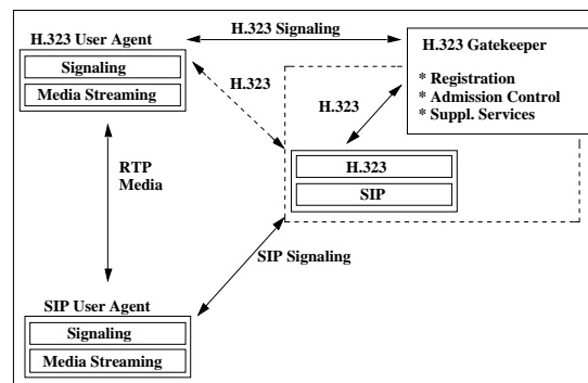
Abbildung 5: SIP-H.323 Gateway
