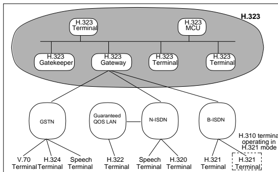
Abbildung 2: H.323 Komponenten
