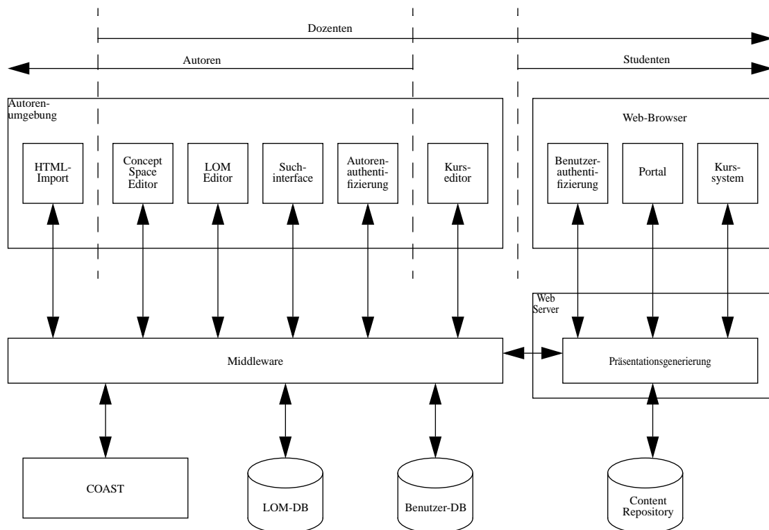
Abbildung 2: Systemarchitektur des kmed -Rahmensystems
