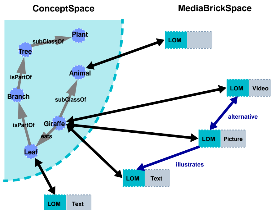
Abbildung 1: ConceptSpace und MediaBrickSpace
