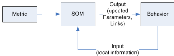
Figure 1. SOM overview.
