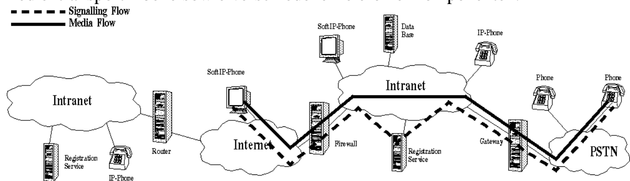
Bild 6 Generisches IP Telefonie Szenario
