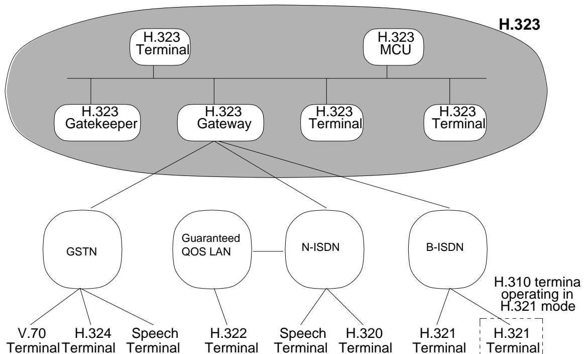
Bild 2 H.323 Komponenten
