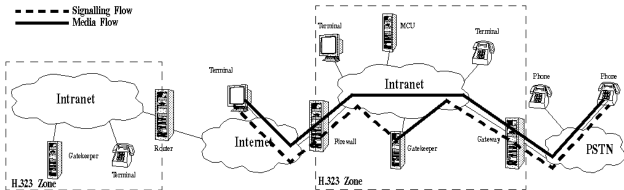
Bild 7 H.323 IP Telefonie Szenario
