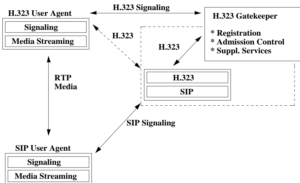
Bild 5 SIP H.323 Gateway
