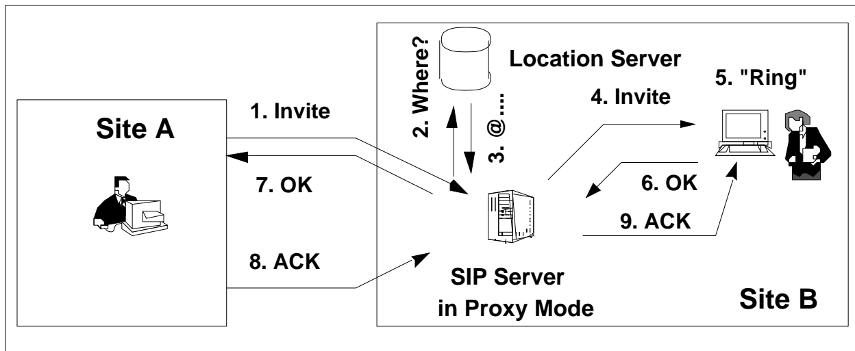
Bild 3 SIP Gesprächsaufbau
