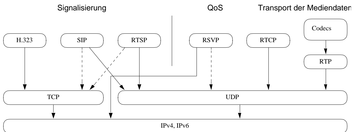
Bild 1 Zusammenwirkung der Protokolle
