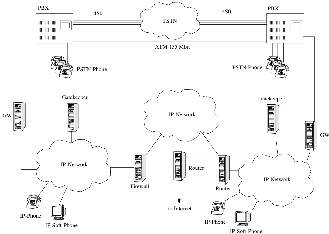
Bild 8 Untersuchtes Test Szenario
